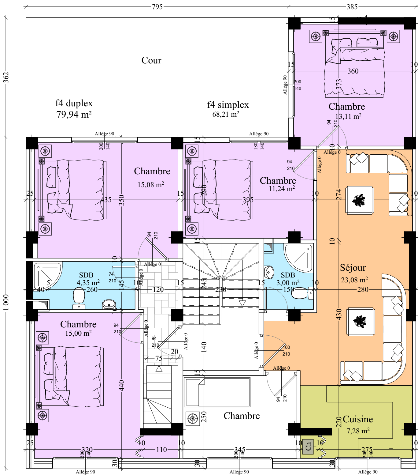
Plan du 1 er étage niv +3,06
