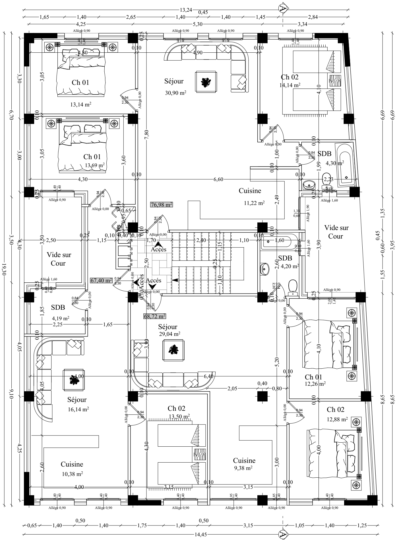
PLAN DU 1er,2eme,3eme ET 4eme ETAGE ECH 1/50
