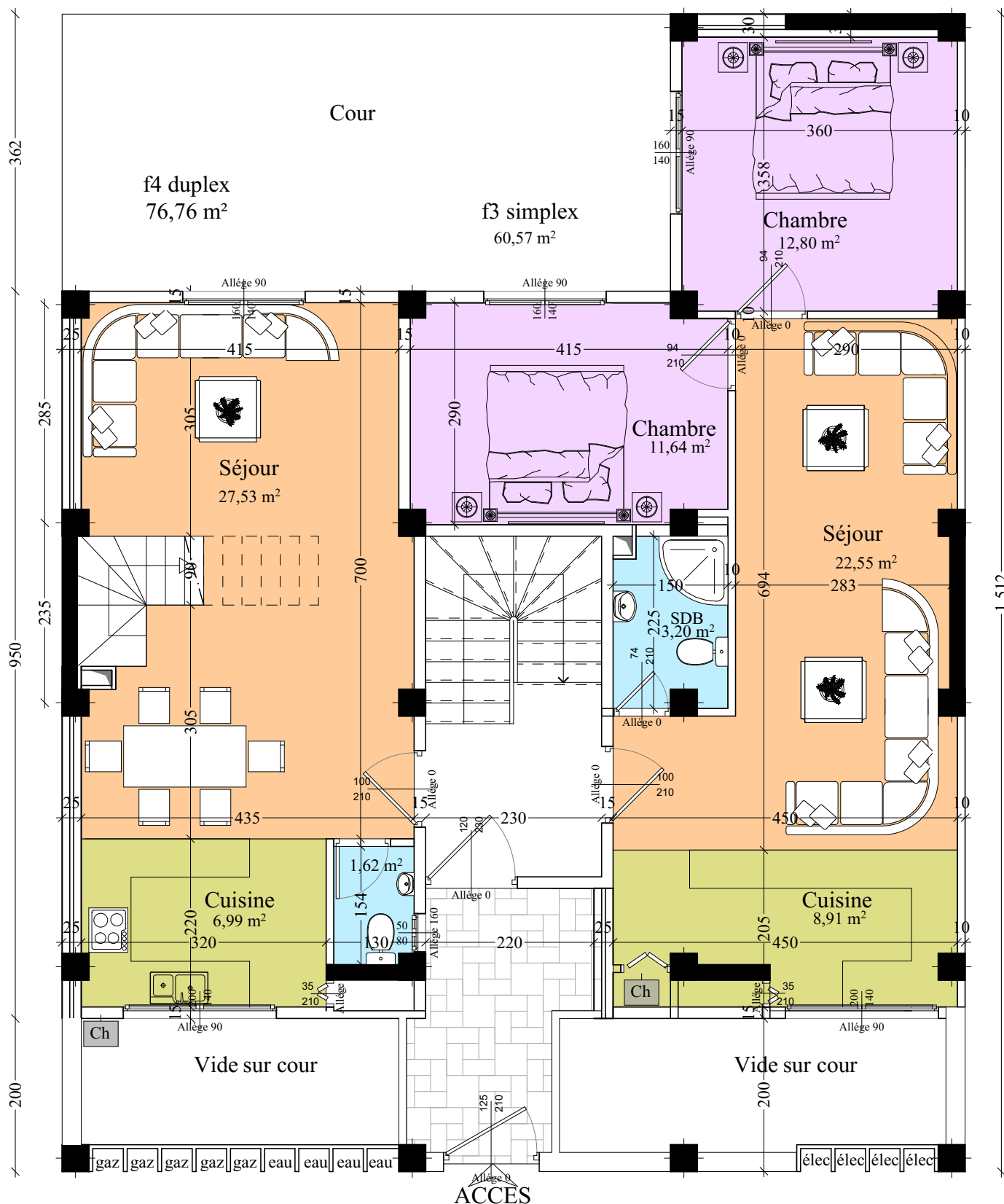
Plan RDC NIV +0,00
