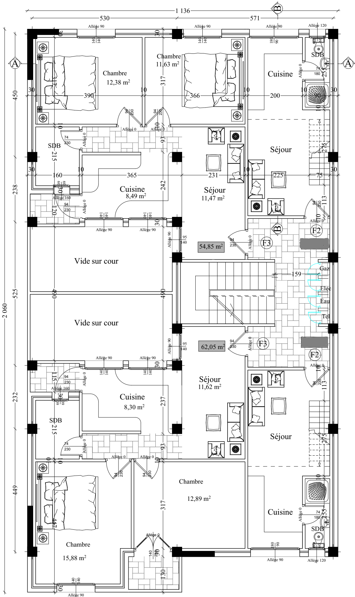
PLAN DU 3 eme ETAGE
