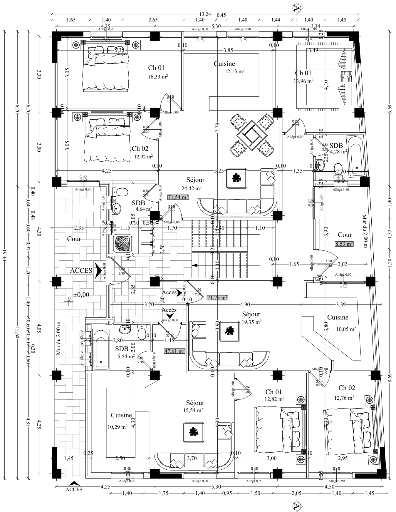
PLAN DU RDC ECH 1/50
